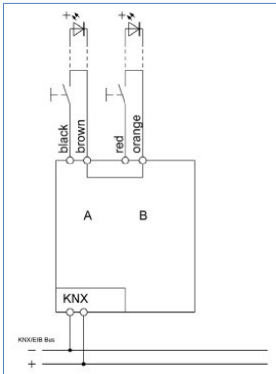
Abbildung 2: Anschlussbeispiel BE0200.01-Ausführung mit 2 Eingängen
