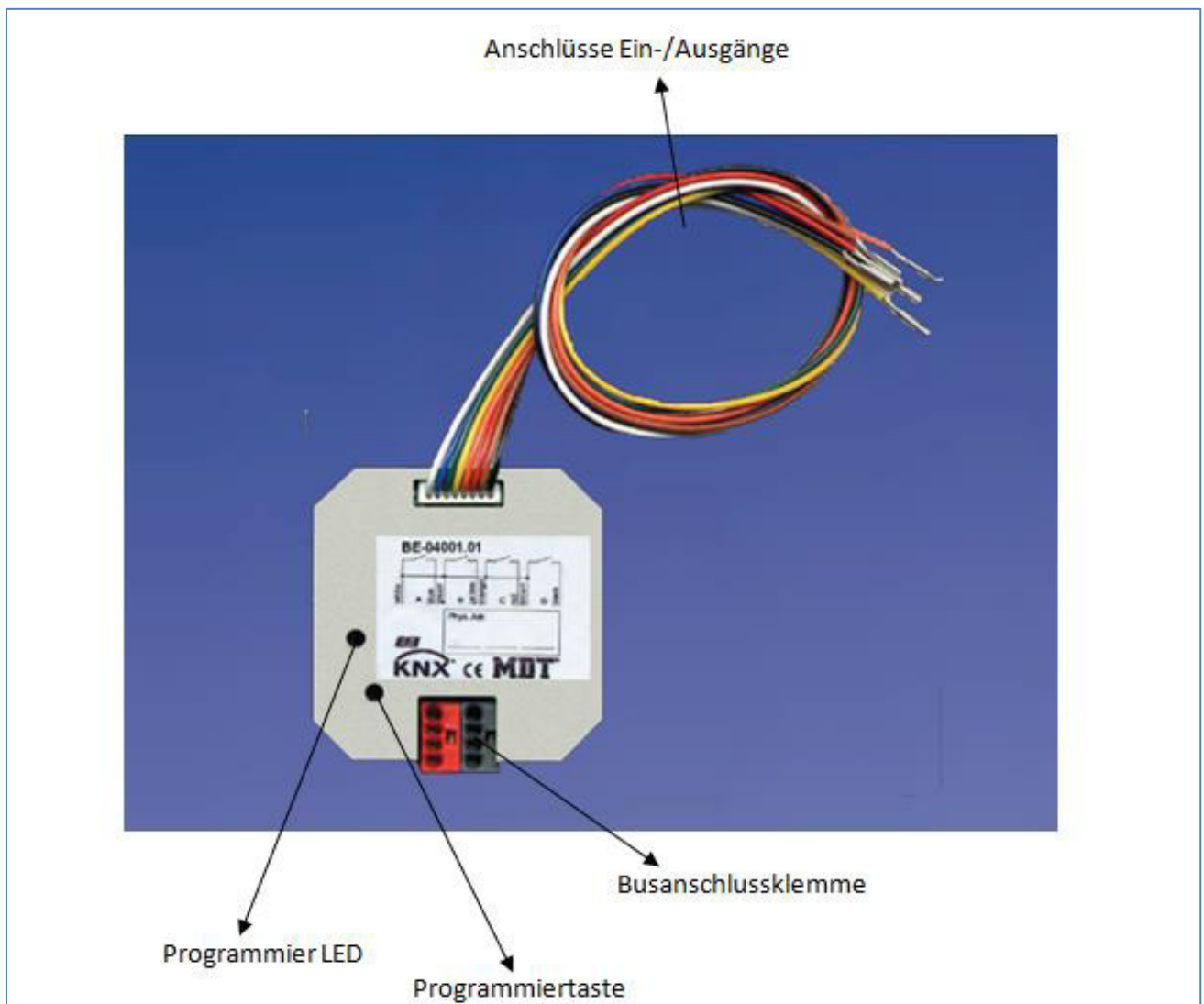
Abbildung 3: Übersicht Hardwaremodul Tasterinterface (hier: BE-0400.01; potentialfrei, 4 fach)
