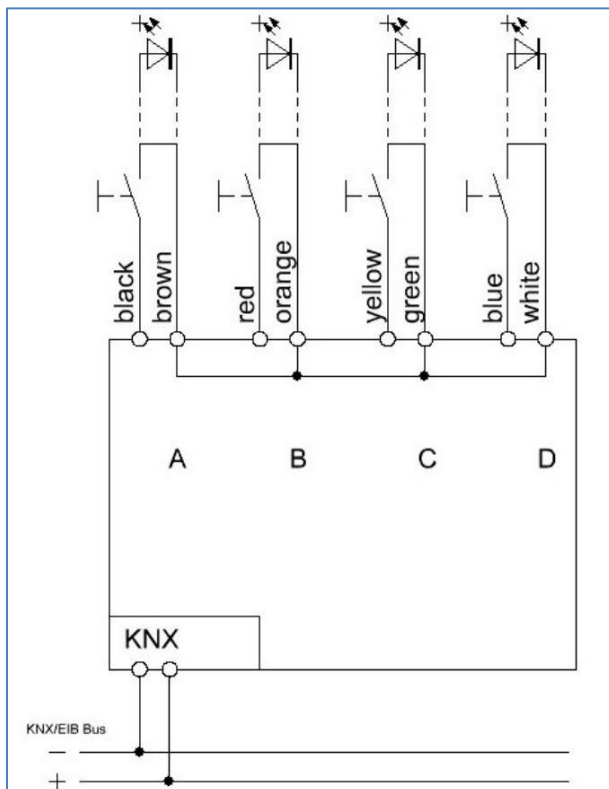
Abbildung 1: Anschlussbeispiel BE0400.01-Ausführung mit 4 Eingängen
